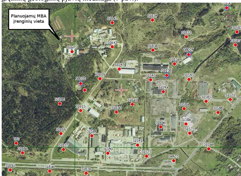
PŪV galimo poveikio žemės gelmėms aspektu yra svarbi viršutinio geologinio pjūvio (iki 100 m nuo žemės paviršiaus) litologinė sudėtis, lemianti gruntinio ir tarpsluoksninio požeminio vandens apsaugotumo nuo antžeminės taršos sąlygas. Nagrinėjamos, Nemuno ir Neries upės apribotos geologinio rajono, terito-
